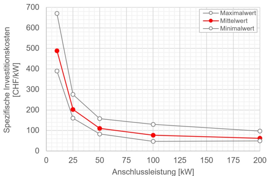
Bild 5.3 Spezifische Investitionskosten in Abhängigkeit der Anschlussleistung für eine Fernwärme-Übergabestation.
