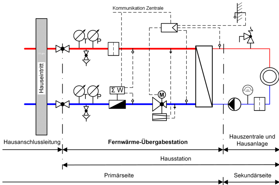
Bild 2.3 Hausanschluss mit indirekter Wärmeübergabe.
