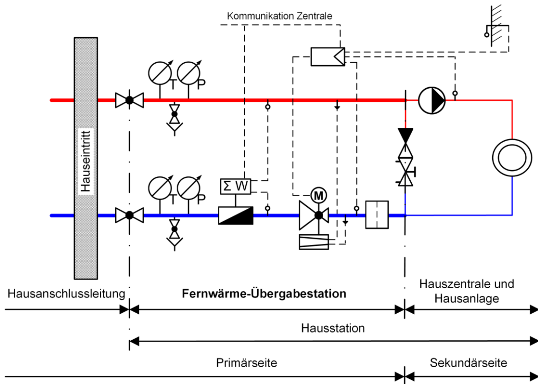
Bild 2.2 Hausanschluss mit direkter Wärmeübergabe.
