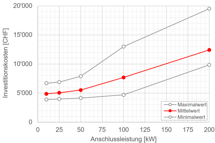
Bild 5.2 Investitionskosten in Abhängigkeit der Anschlussleistung für eine Fernwärme-Übergabestation.
