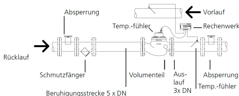
Bild 4.2 Installation Wärmezähler (Quelle: WDV-Molliné GmbH).
