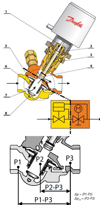
Bild 4.1 Schnitt durch ein differenzdruckunabhängiges Regelventil (Bildquelle: Danfoss AB-QM). Das Ventil besteht aus einem Differenzdruckregler (gelb) und einem Regelventil (orange).
