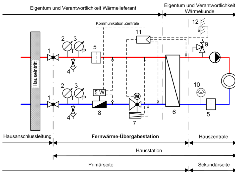
Bild 5.1 Minimalanforderung Fernwärme-Übergabestation.
