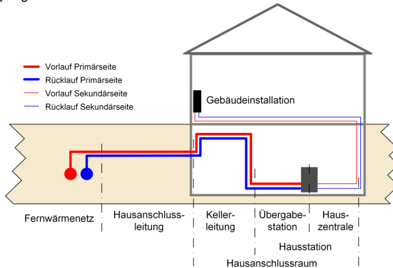
Bild 2.1 Übersicht zum Hausanschluss.
