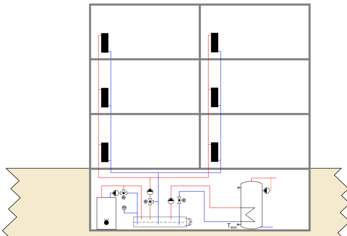
Bild 9.1 Fallbeispiel: Ausgangslage bei Interesse für einen Fernwärmeanschluss.
