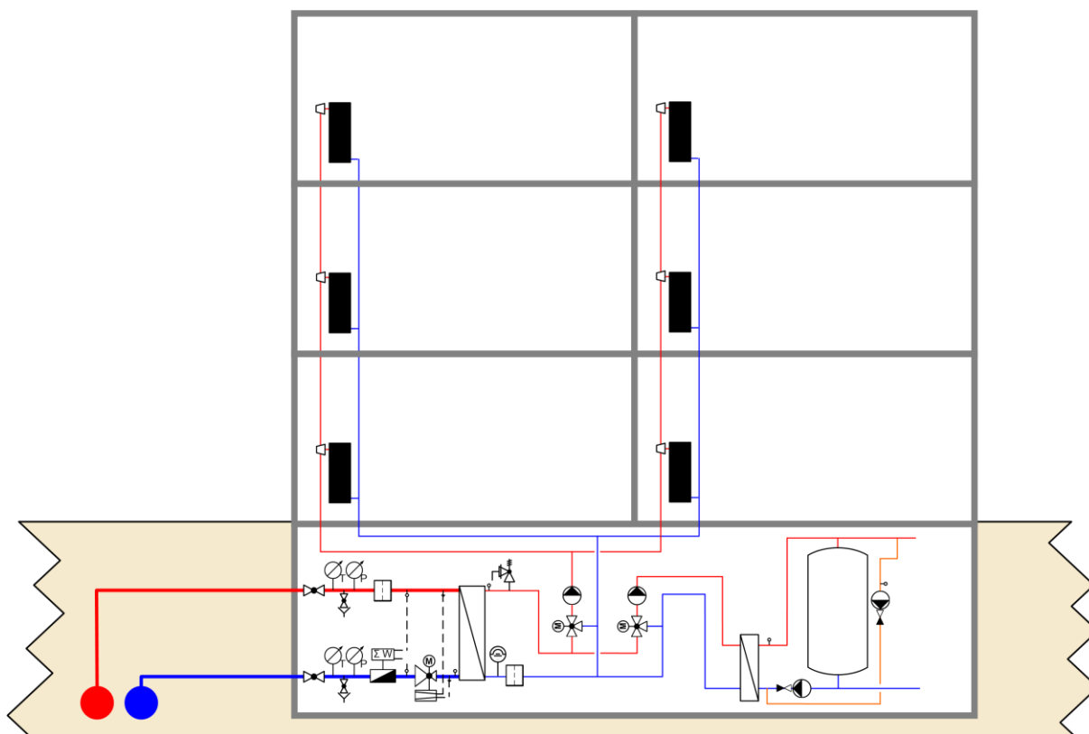
Bild 9.3 Fallbeispiel: Anschluss an Fernwärmenetz und Umbau Sekundärseite.
